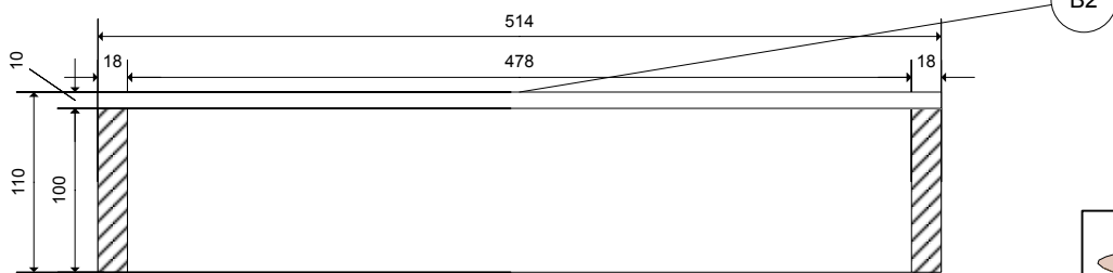
Doorsnede A - B
